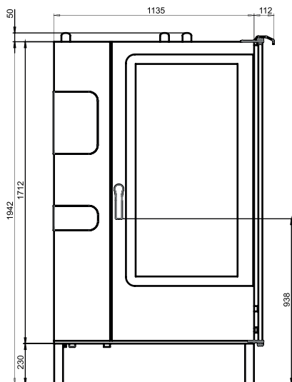
Pohled zepředu
