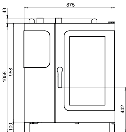
Pohled zepředu
