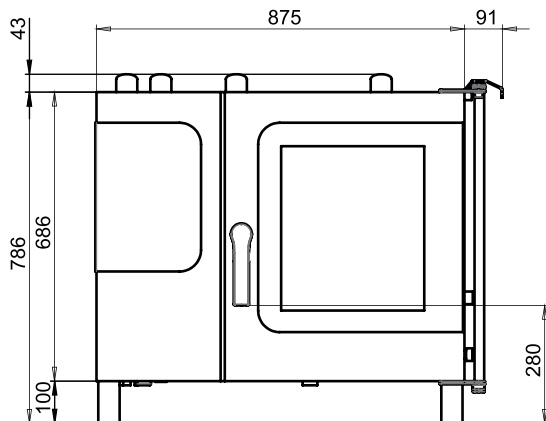
Pohled zepředu
