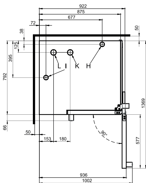
Pohled shora se vzdálenostmi od stěny
