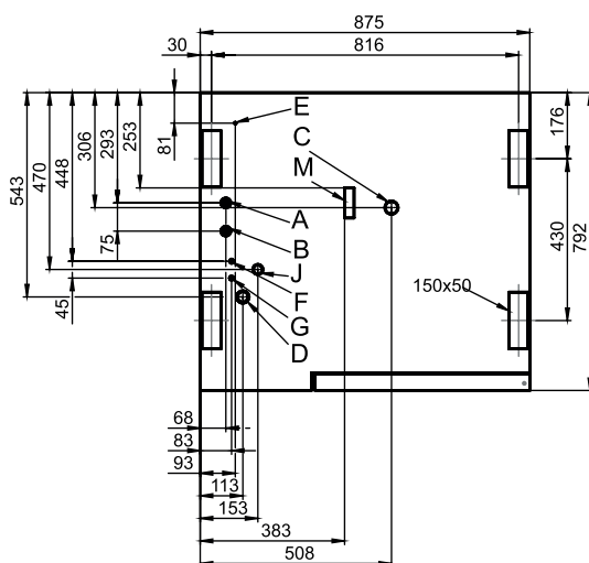
Pozice přípojek dna přístroje
