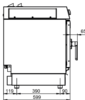
Pozice přípojek dna přístroje
