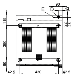
Pozice přípojek dna přístroje
