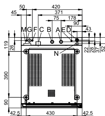
Pozice přípojek dna přístroje
