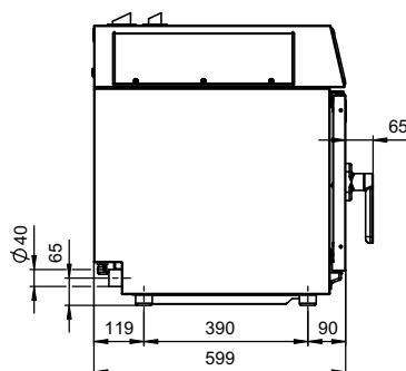
Pohled ze strany
