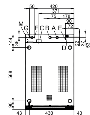
Pozice přípojek dna přístroje
