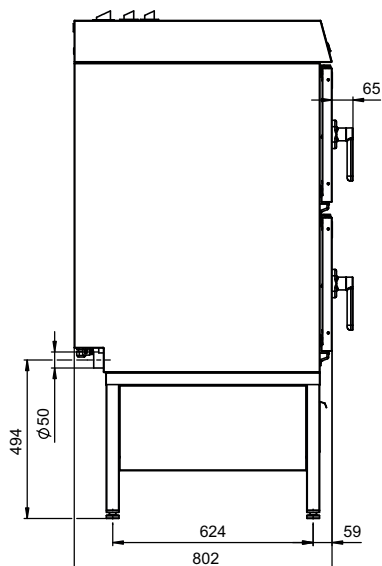
Pozice přípojek dna přístroje
