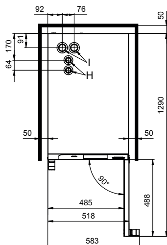
Pohled shora se vzdálenostmi od stěny
