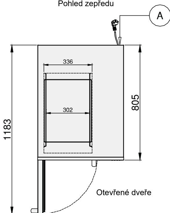
Pohled zepředu
