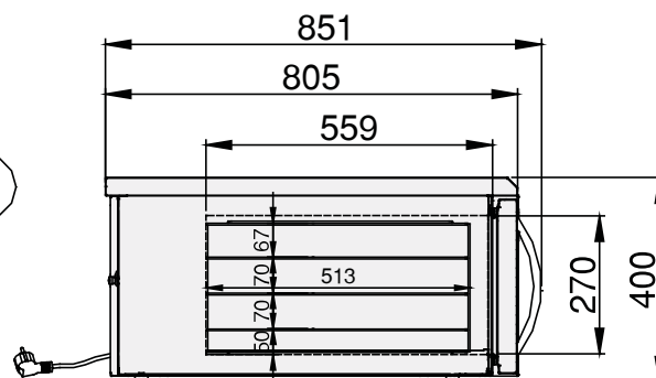
Boční pohled
