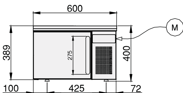
Pohled zepředu
